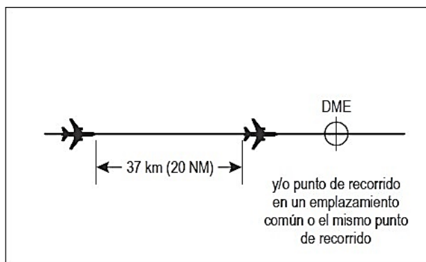
Figura 5-22. Separación de 20 NM basada en DME y/o en GNSS entre aeronaves por la misma derrota y al mismo nivel véase [5.4.2.3.3.1 a)]
