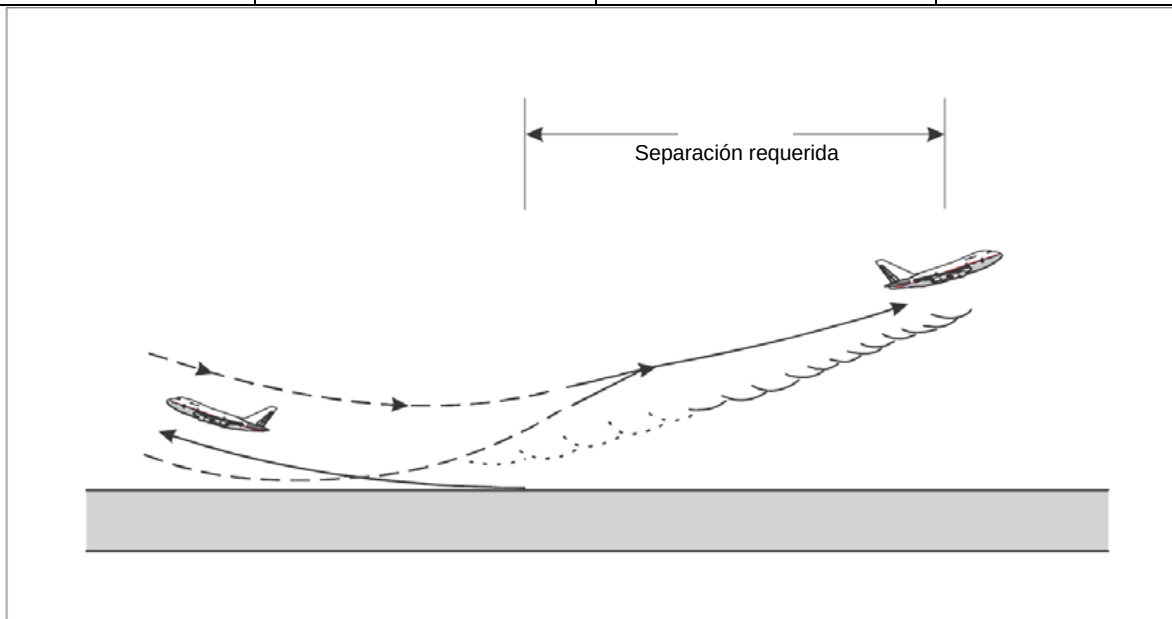
Figura 5-45. Separación por estela turbulenta para despegue en sentidos opuestos [véanse 5.8.5.1 a) y 5.8.5.2 a)]
