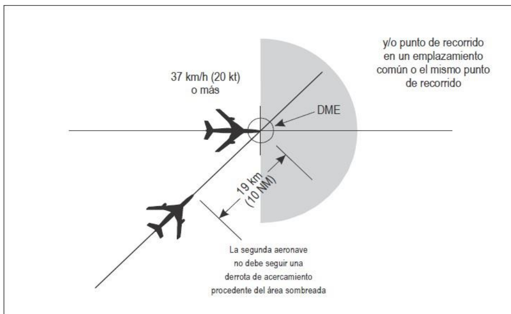
Figura 5-24B. Separación de 10 NM basada en DME y/o en GNSS entre aeronaves por derrota que se cruzan y al mismo nivel (véase 5.4.2.3.3.2)
