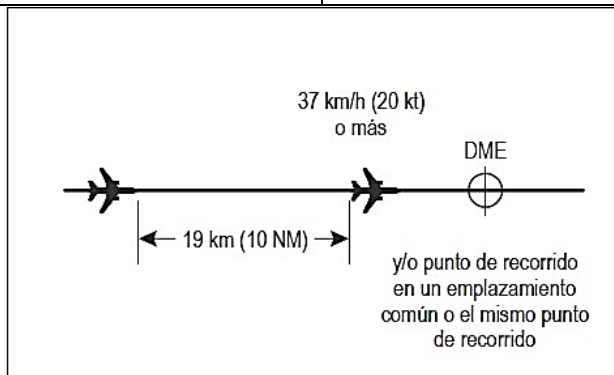
Figura 5-23. Separación de 10 NM basada en DME y/o en GNSS entre aeronaves por la misma derrota y al mismo nivel [véase 5.4.2.3.3.1 b)]
