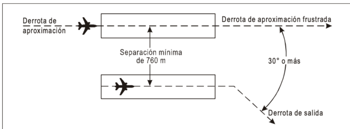
Figura 6-7. Operaciones paralelas segregadas [vease 6.7.3.6.1 b)]
