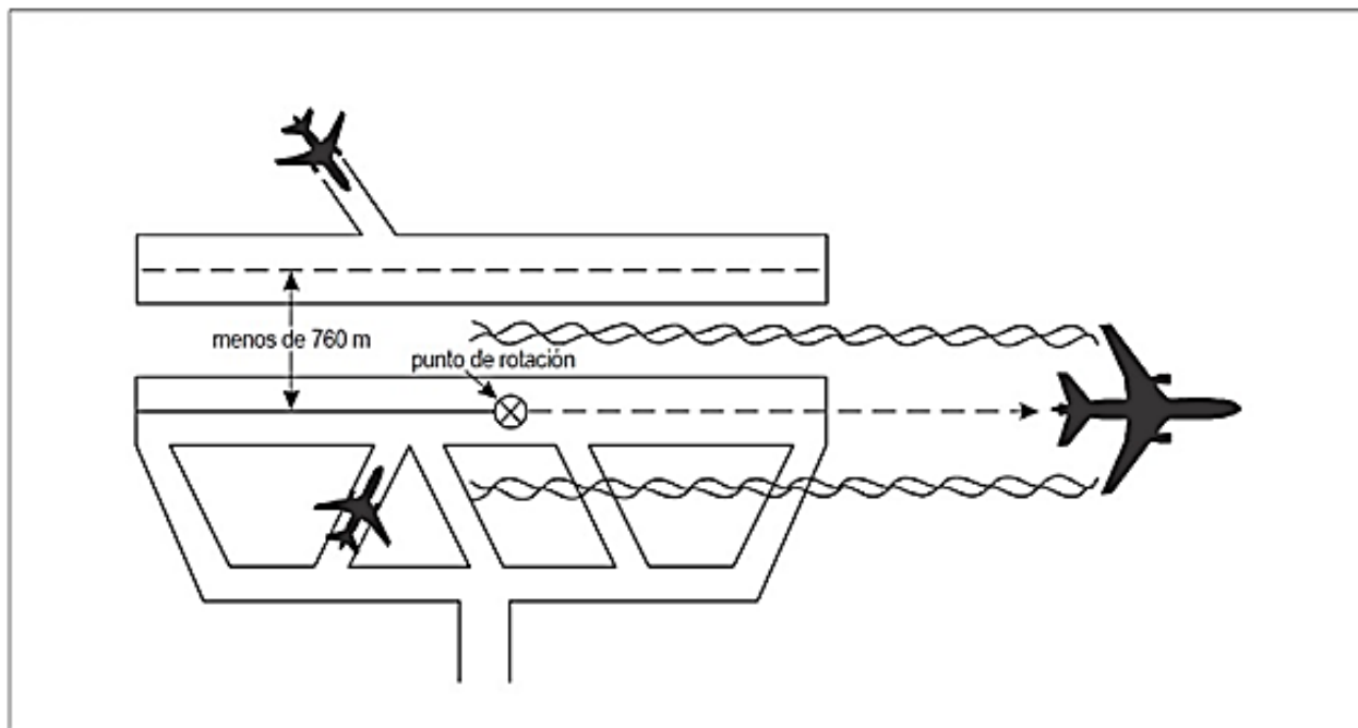
Figura 5-44. Separación por estela turbulenta para la aeronave que sigue (veáanse 5.8.3.3 y 5.8.3.4)
