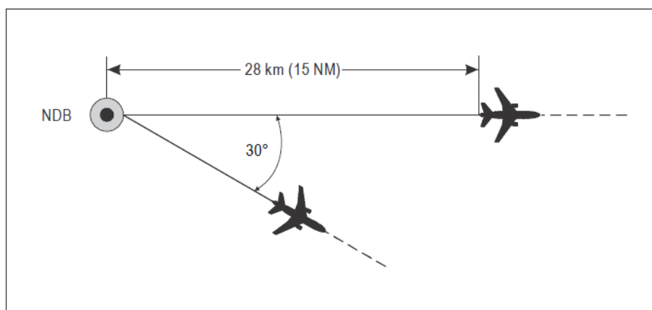
Figura 5-5. Separación utilizando el mismo NDB (véase 5.4.1.2.1.2 b)
