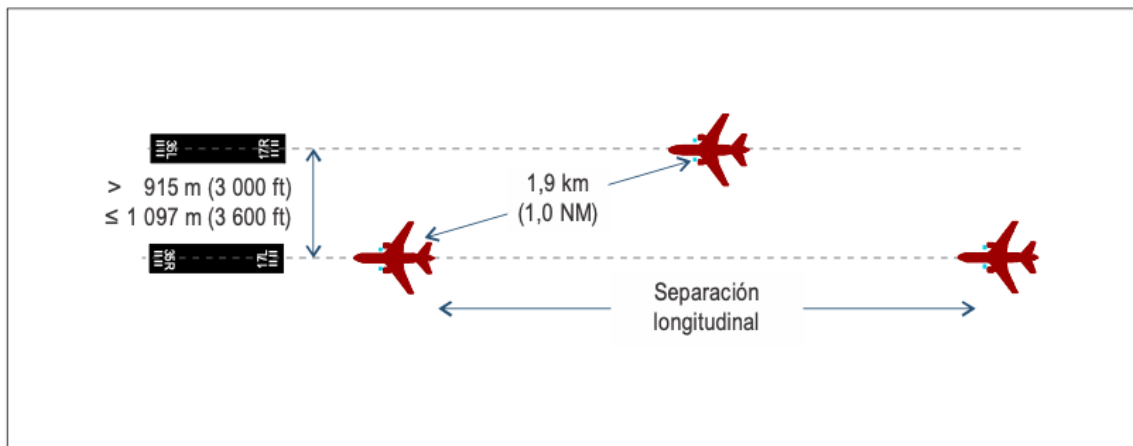
Figura 6-5. Separación diagonal para una distancia entre ejes mayor que 915 m pero menor o igual a 1.097 m
