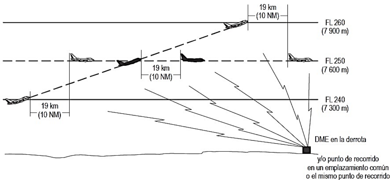
Figura 5-25A. Separación de 10 NM basada en DME y/o en GNSS entre aeronaves que ascienden y por la misma derrota [véase 5.4.2.3.4.1 c)]
