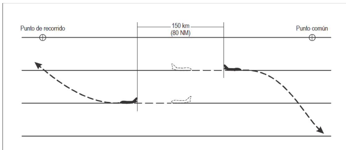
Figura 5-28. Separación de 80 NM basada en RNAV entre aeronaves por derrota opuestas (véase 5.4.2.5.7)
