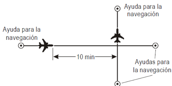
Figura 5-15. Separación de 10 minutos entre aeronaves por derrota que se cruzan y al mismo nivel [véase 5.4.2.2.1.2 b)]
