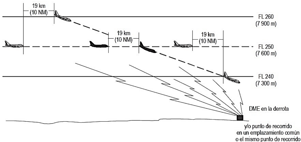
Figura 5-25B. Separación de 10 NM basada en DME y/o en GNSS entre aeronaves que descienden y por la misma derrota [véase 5.4.2.3.4.1 c)]
