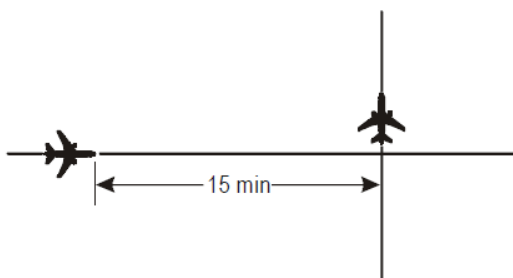
Figura 5-14. Separación de 15 minutos entre aeronaves por derrota que se cruzan y al mismo nivel [véase 5.4.2.2.1.2 a)]
