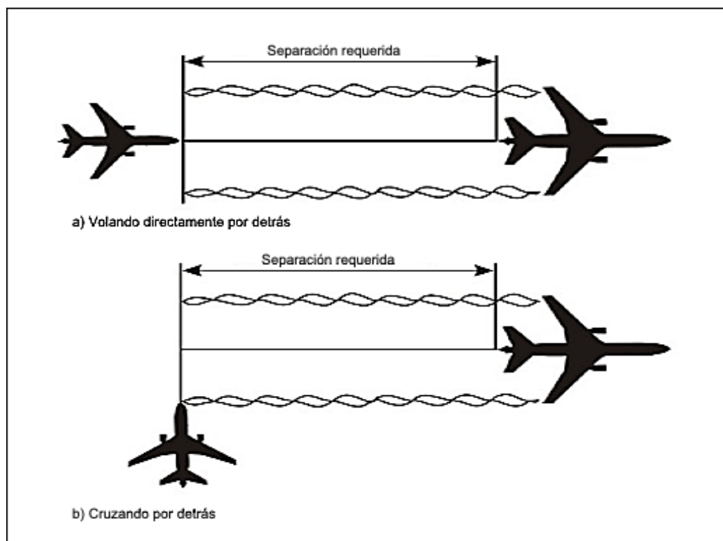
Figura 8-1. Vuelo directamente por detrás o cruce por detrás (véanse 8.7.3.4. y 8.7.3.5)
