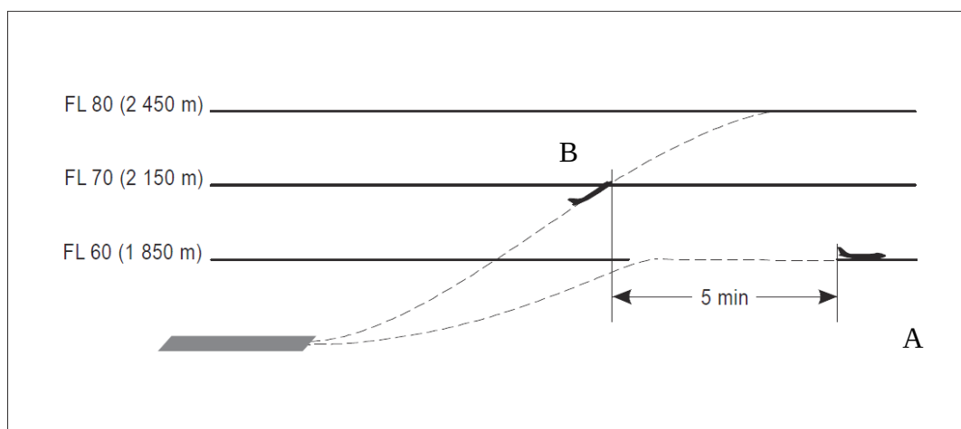
Figura 5-39. Separación de cinco minutos entre aeronaves que salen siguiendo la misma derrota (véase 5.6.3)
