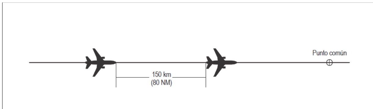
Figura 5-26. Separación de 80 NM basada en RNAV entre aeronaves al mismo nivel [véase 5.4.2.5.5 b)]
