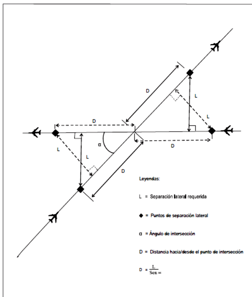
Figura 5-6 Puntos de separación lateral (véase 5.4.1.2.1.7)
