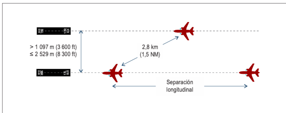
Figura 6-4. Separación diagonal para una distancia entre ejes mayor que 1.097 m, pero menor o igual a 2.529 m
