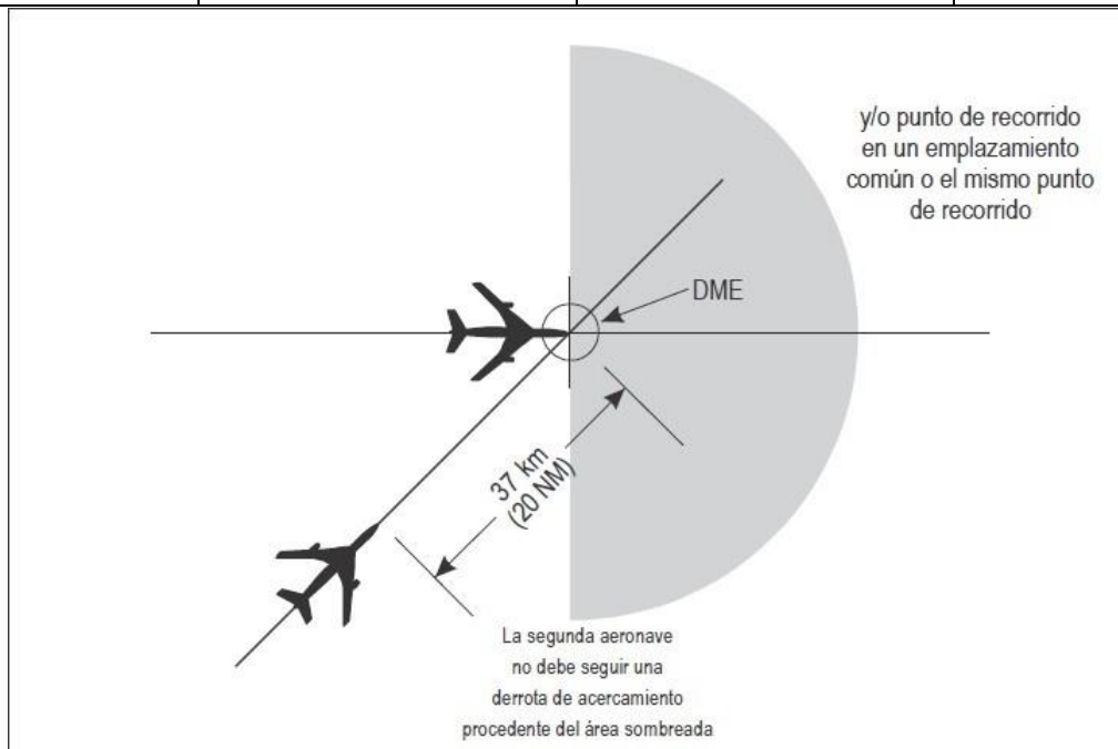
Figura 5-24A. Separación de 20 NM basada en DME y/o en GNSS entre aeronaves por derrota que se cruzan y al mismo nivel (véase 5.4.2.3.3.2)
