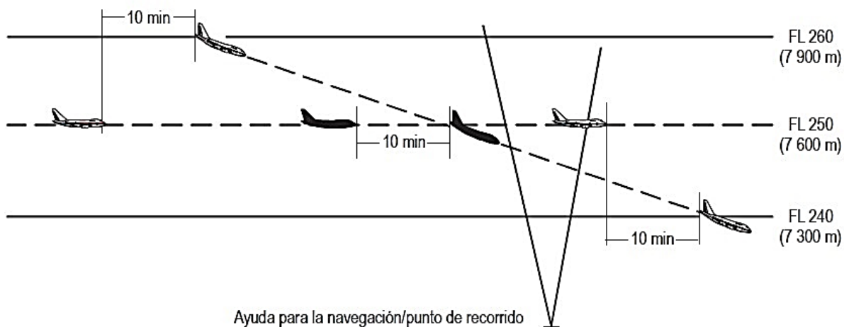
Figura 5-17B. Separación de 10 minutos entre aeronaves que descienden y por la misma derrota [véase 5.4.2.2.2.1 b)]
