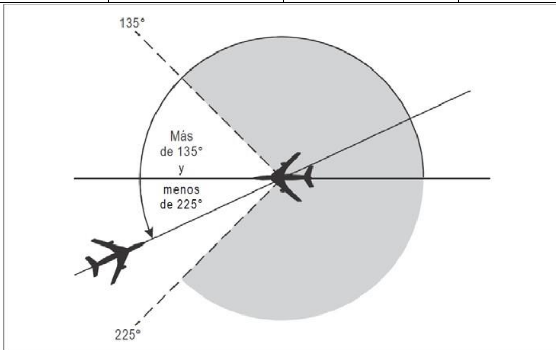
Figura 5-8. Aeronaves por derrotas opuestas (véase 5.4.2.1.5 b)
