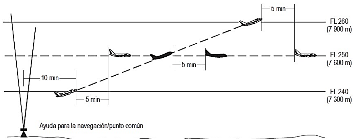
Figura 5-18A. Separación de 5 minutos entre aeronaves que ascienden y por la misma derrota [véase 5.4.2.2.2.1 c)]
