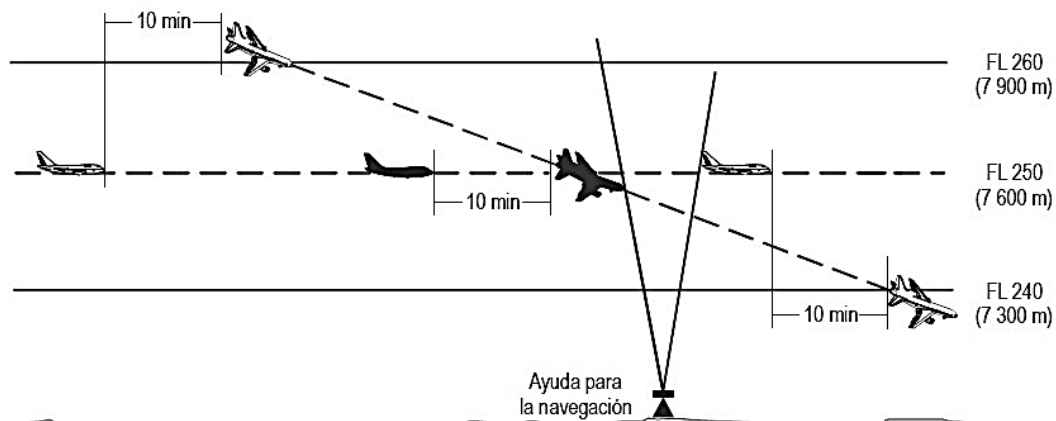
Figura 5-20B. Separación de 10 minutos entre aeronaves que descienden y por derrotas que se cruzan [véase 5.4.2.2.2.2 b)]
