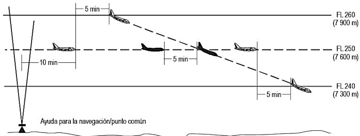
Figura 5-18 B. Separación de 5 minutos entre aeronaves que descienden y por la misma derrota [véase 5.4.2.2.2.1 c) 2)]
