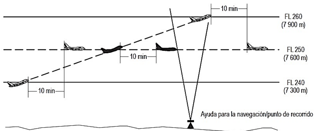
Figura 5-17A. Separación de 10 minutos entre aeronaves que ascienden y por la misma derrota [véase 5.4.2.2.2.1 b)]
