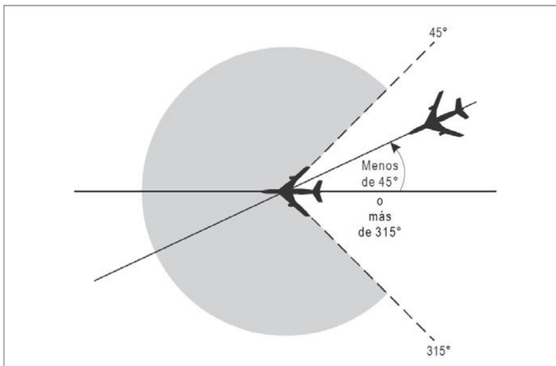
Figura 5-7. Aeronaves por la misma derrota (véase 5.4.2.1.5 a)
