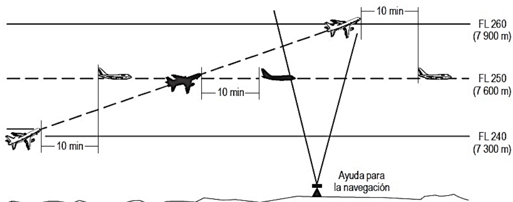
Figura 5-20A. Separación de 10 minutos entre aeronaves que ascienden y por derrotas que se cruzan [véase 5.4.2.2.2.2 b)]
