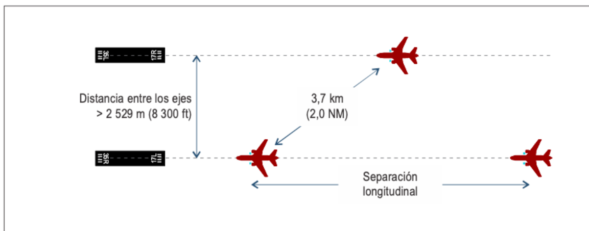
Figura 6-3. Separación diagonal para una distancia entre ejes mayor que 2.529 m
