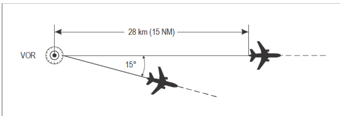
Figura 5-4. Separación utilizando el mismo VOR (véase 5.4.1.2.1.2 a)
