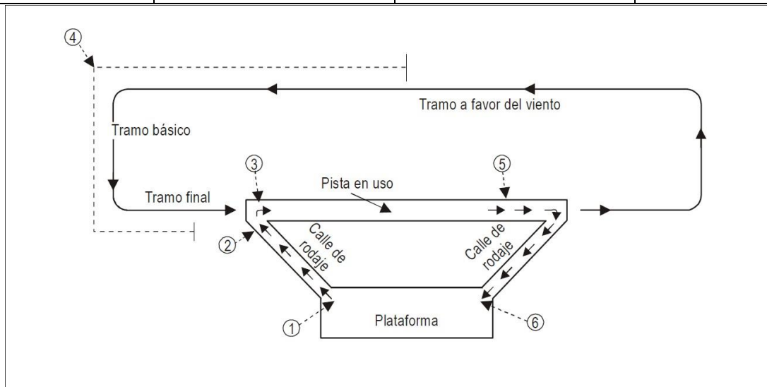
Figura 7-1. Posiciones designadas de las aeronaves desde un punto de vista de la torre de control del aeródromo
